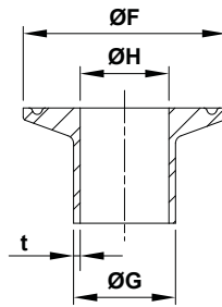
DIN 32676
